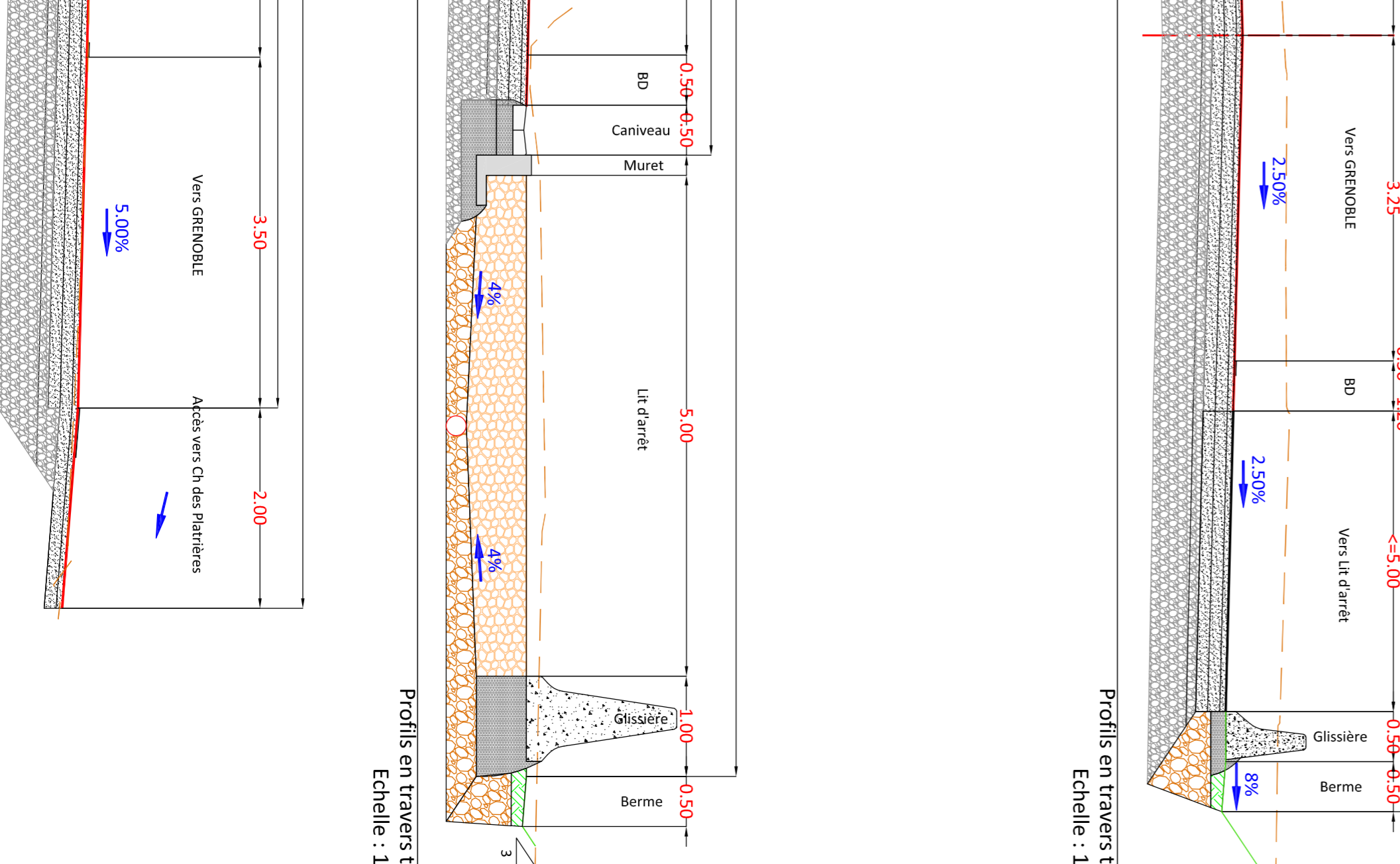
Profil en travers type 1 Profil en travers type 2 Profil en travers type 3 Profil en travers type 4 Echelle : 1/50
